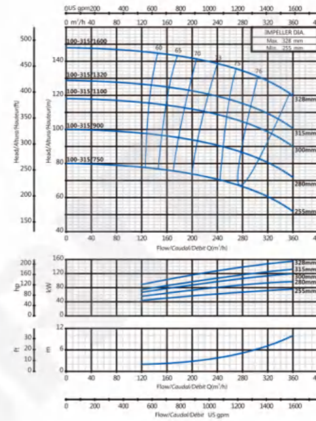
100-315
