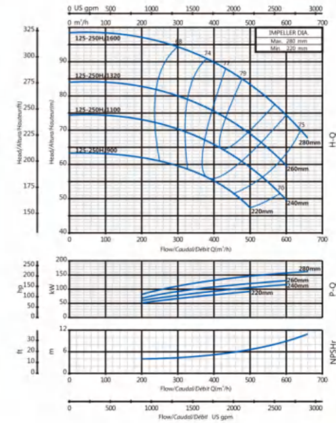
125-250H
