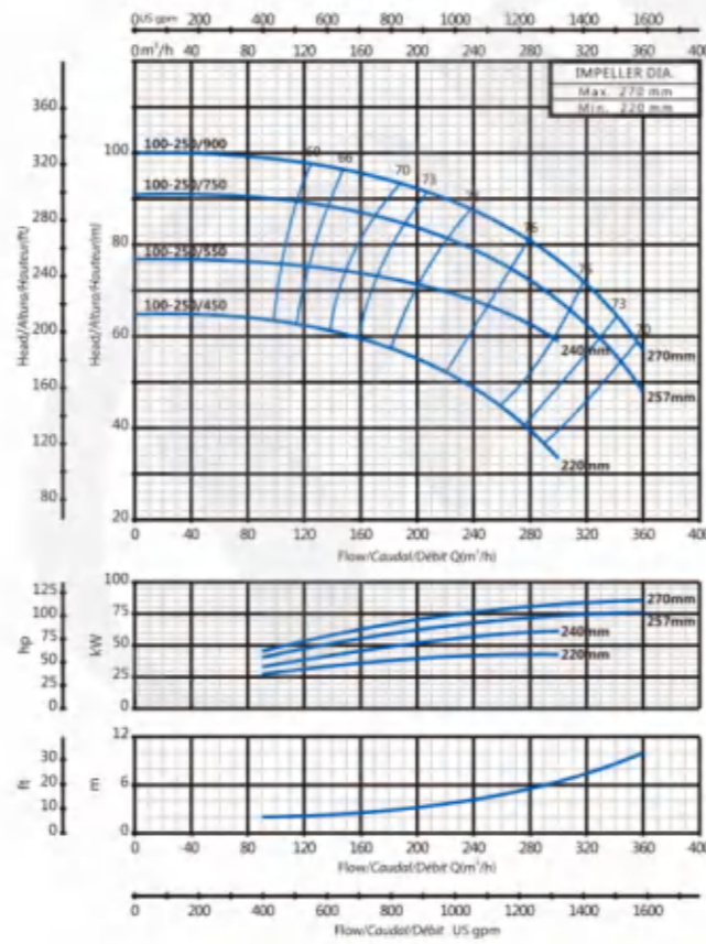
100-250
