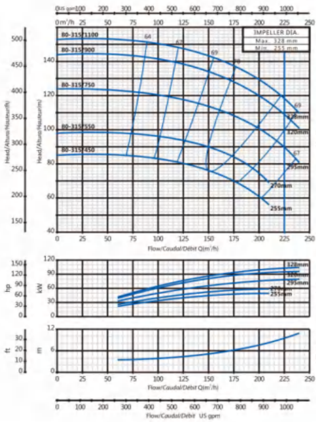
80-315
