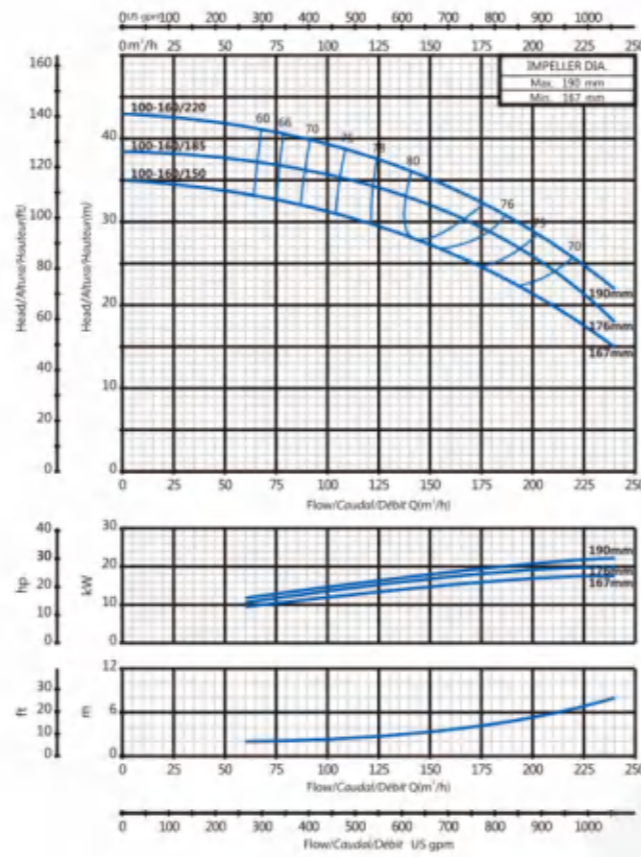
100-160
