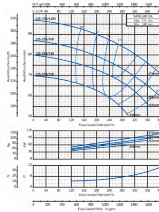
125-250
