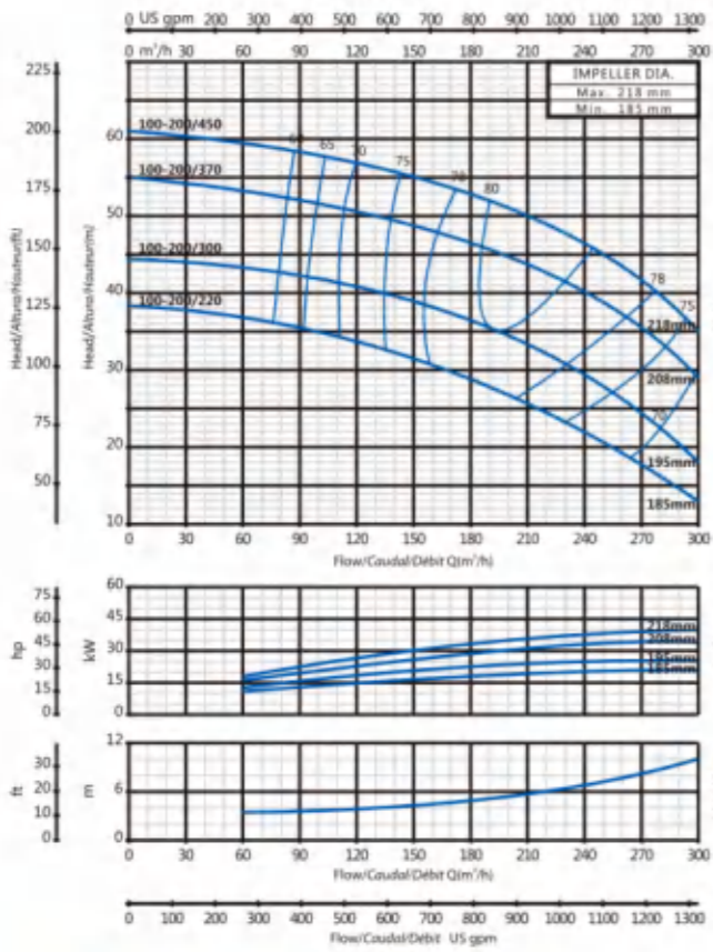
100-200
