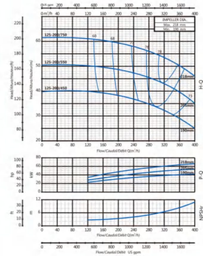
125-200
